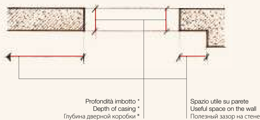
Pianta - Plan - План
